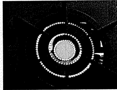
QUEIMADOR CHAMA TRIPLA FRONTAL Chama interna com Ø 50mm e potência de 756 kcal/h Chama dupla externa com Ø 150mm e potência de 3.334 kcal/h.
